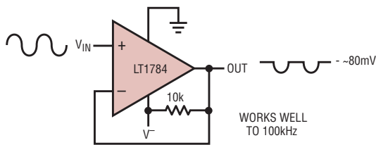
Negative Rectifier
